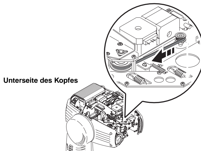
Bild 18: Prisma nach vorne bewegen
