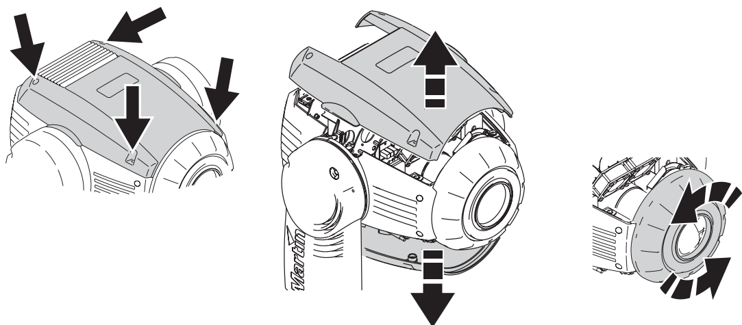
Bild 16: Entfernen der Kopfabdeckungen und der Frontlinse
