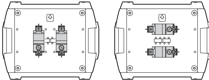
Bild 6: Montagepositionen der Klemmadapter
