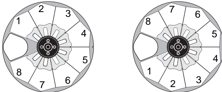
Bild 7: Filterpositionen, Rad 1 (links) und Rad 2 (rechts), von der Frontlinse gesehen
