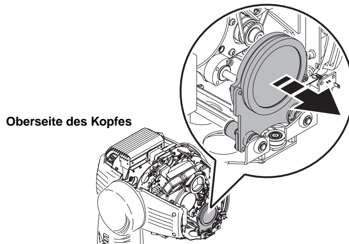
Bild 17: Fokusschlitten nach vorne bewegen
