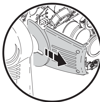
Bild 23: Austauschen der Luftfilter
