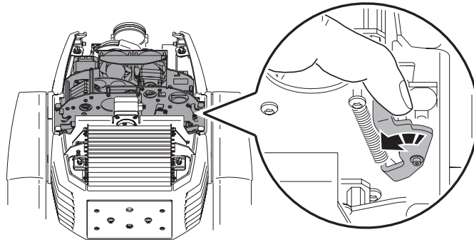
Bild 20: Verriegelungen des Gobomoduls
