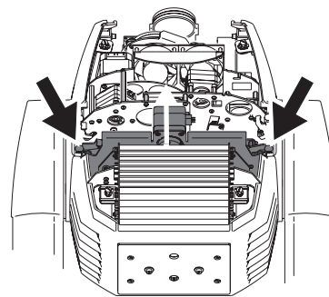
Bild 21: Verriegelungen des Dimmermoduls
